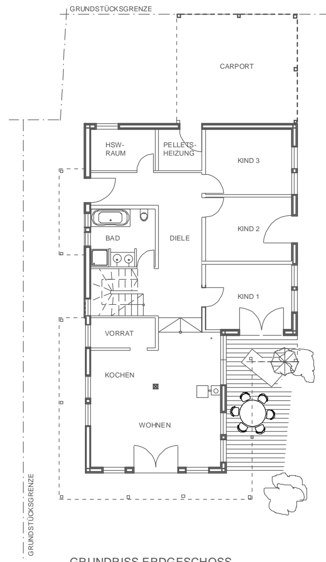
GRUNDRISS ERDGESCHOSS
