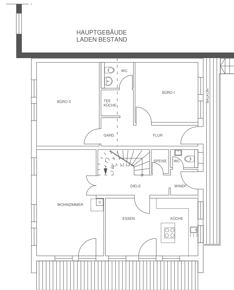
GRUNDRISS 1. OBERGESCHOSS
